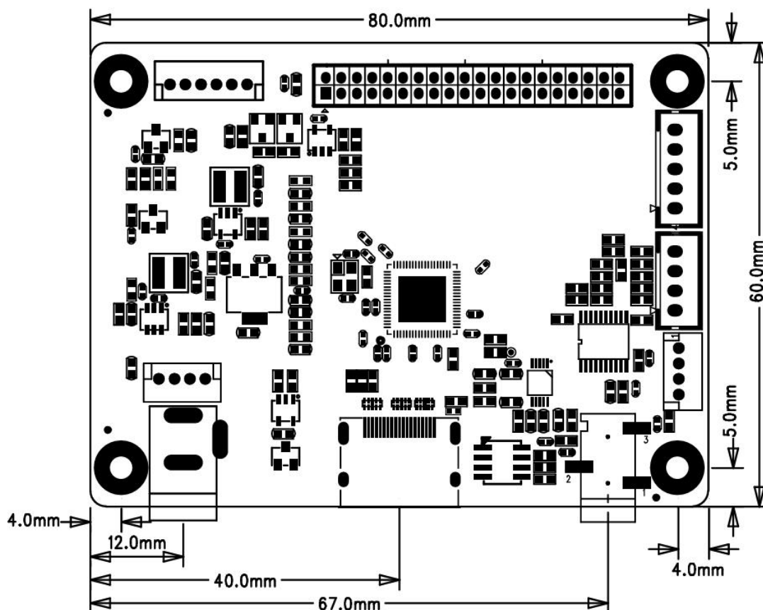
图 8 安装尺寸
