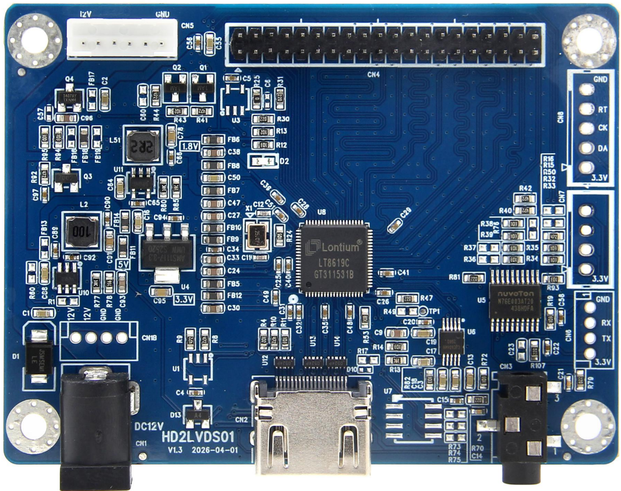
图 1. 板卡 (8x6cm)
