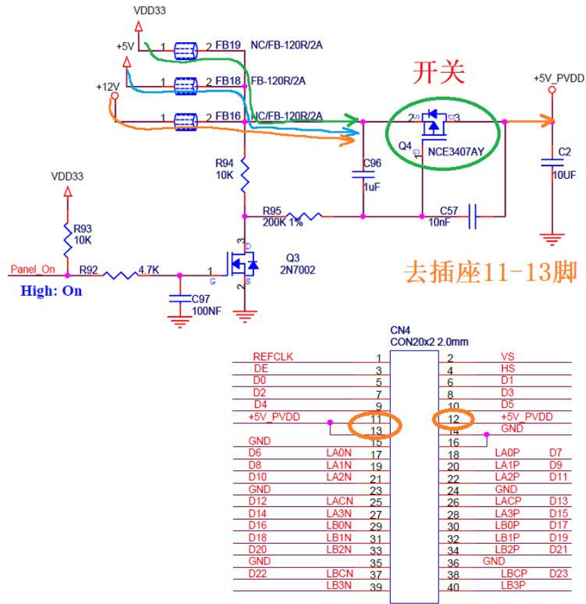
图 6 屏电输出电路
