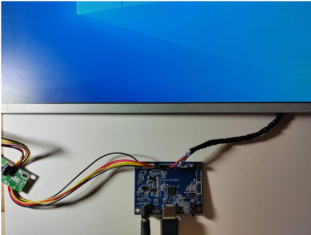
图 10 连接方式 2
