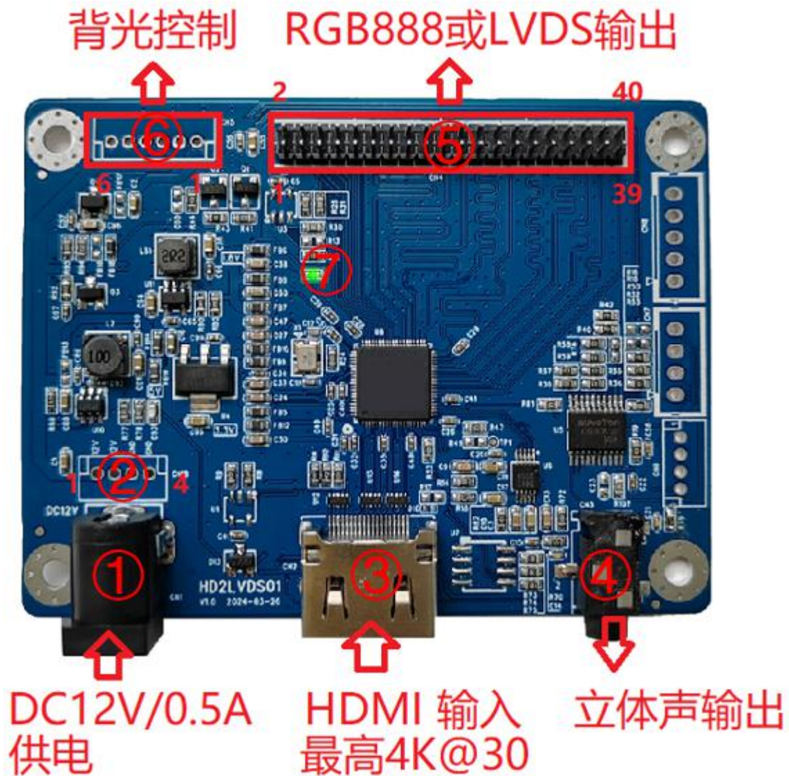
图 2. 接口
