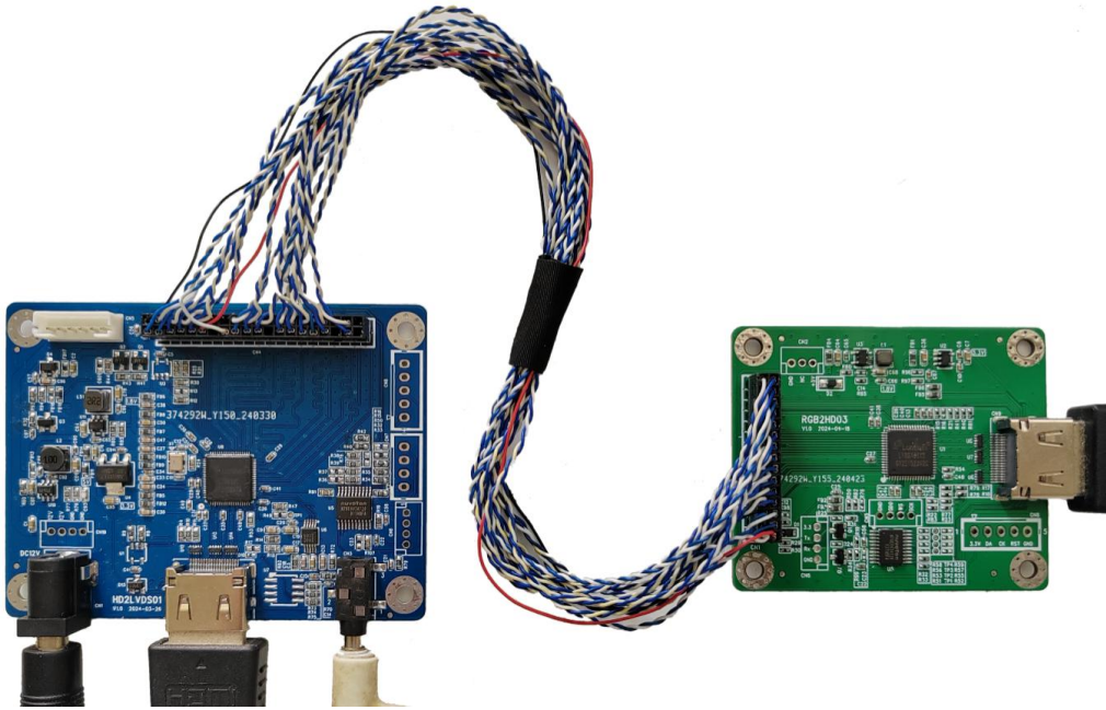
图 9 连接方式 1
